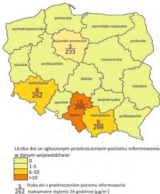
Ryc. 1.3. Przypadki przekroczeń poziomu informowania (24h 200 µg/m 3 ) dla pyłu zawieszonego PM10 w 2016 roku w poszczególnych województwach
