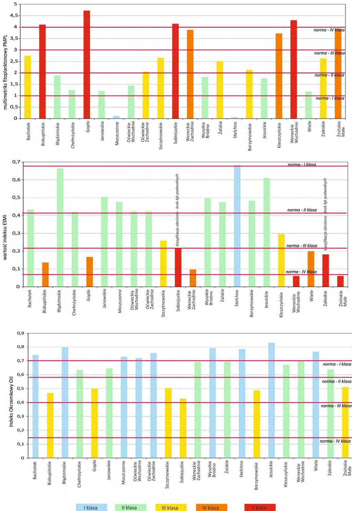
Ryc. 2.5. Klasyfikacja wskaźników biologicznych w jeziorach województwa kujawsko-pomorskiego badanych w 2016 roku
